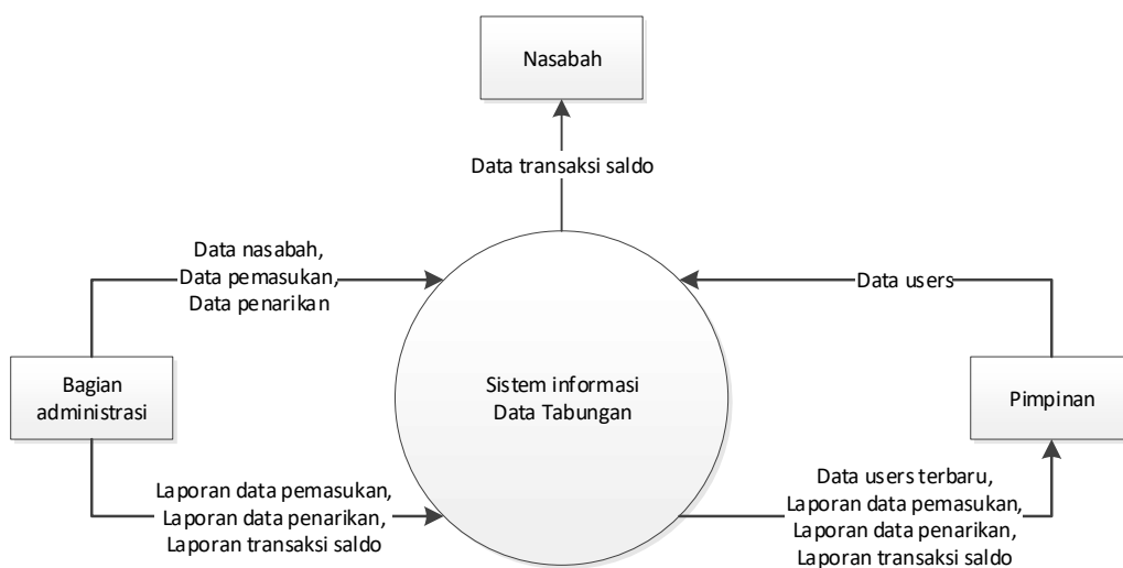
Gambar 3. Diagram konteks
